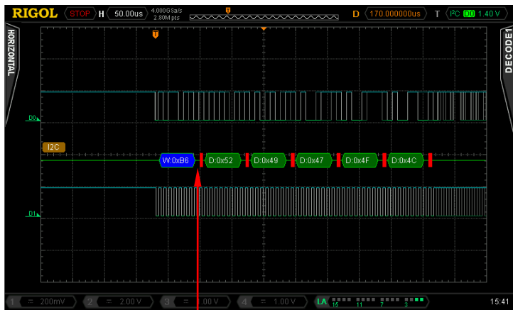
ACK=1
